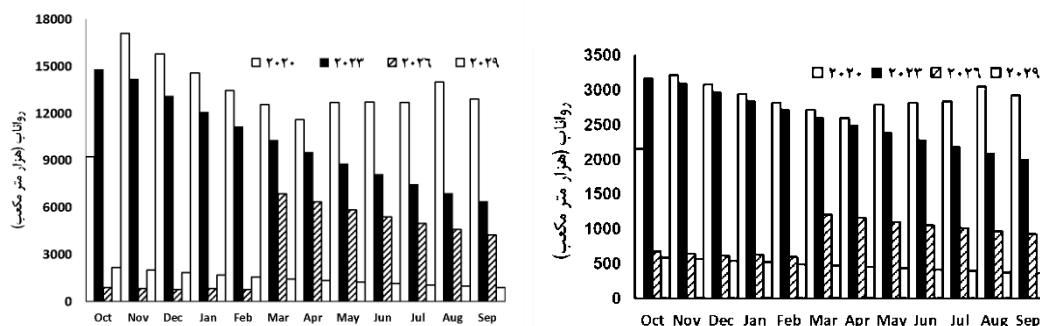
شکل ۶: مقایسه رواناب شبیه‌سازی شده در مقطع‌های زمانی مختلف برای دوره‌های آبی حوزه یامچی و نیر تحت سناریوی A1B
