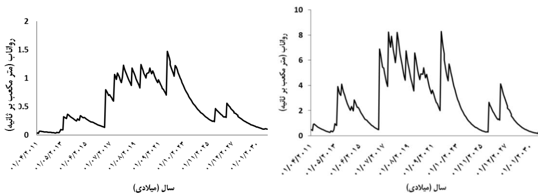
شکل ۵: پیش‌بینی رواناب برای دوره آبی ایستگاه هیدرومتری یامچی و نیر
