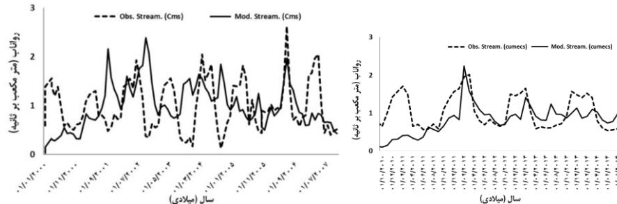
شکل ۴: شبیه‌سازی جریان ماهانه حوضه نیر در دوره واسنجی و اعتبارسنجی توسط مدل IHACRES
