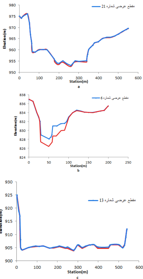
شکل (۴): نتایج حاصل از شبیه سازی شبه غیر ماندگار برای مقاطع عرضی انتخابی
