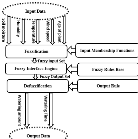
شکل (۲): بلوک دیاگرام سیستم منطقی فازی
