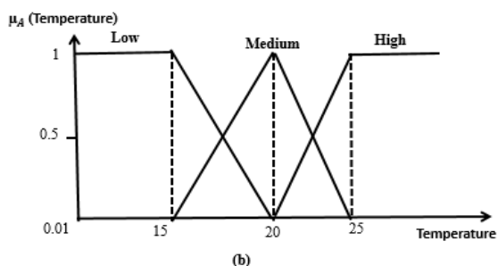
شکل (۳): توابع عضویت برای متغیرهای ورودی
