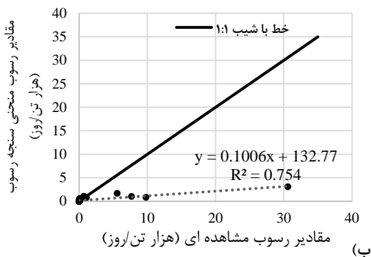
شکل (۱۱): مقادیر مشاهده‌ای و پیش‌بینی مدل برای مدل‌های الگوریتم ژنتیک (الف) و منحنی سنجیده رسوب (ب) برای داده‌های آزمون ایستگاه باغ‌عباسی
