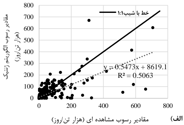
شکل (۱۰): مقادیر مشاهده‌ای و پیش‌بینی مدل برای مدل‌های الگوریتم ژنتیک (الف) و منحنی سنجیده رسوب (ب) برای داده‌های آزمون ایستگاه قزاقلی
