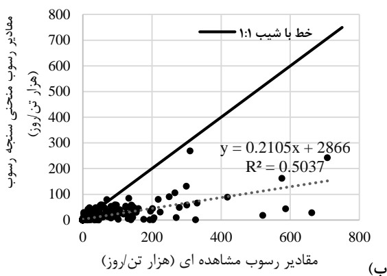
شکل (۱۰): مقادیر مشاهده‌ای و پیش‌بینی مدل برای مدل‌های الگوریتم ژنتیک (الف) و منحنی سنجیده رسوب (ب) برای داده‌های آزمون ایستگاه قزاقلی
