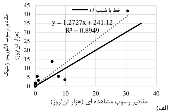
شکل (۱۱): مقادیر مشاهده‌ای و پیش‌بینی مدل برای مدل‌های الگوریتم ژنتیک (الف) و منحنی سنجیده رسوب (ب) برای داده‌های آزمون ایستگاه باغ‌عباسی
