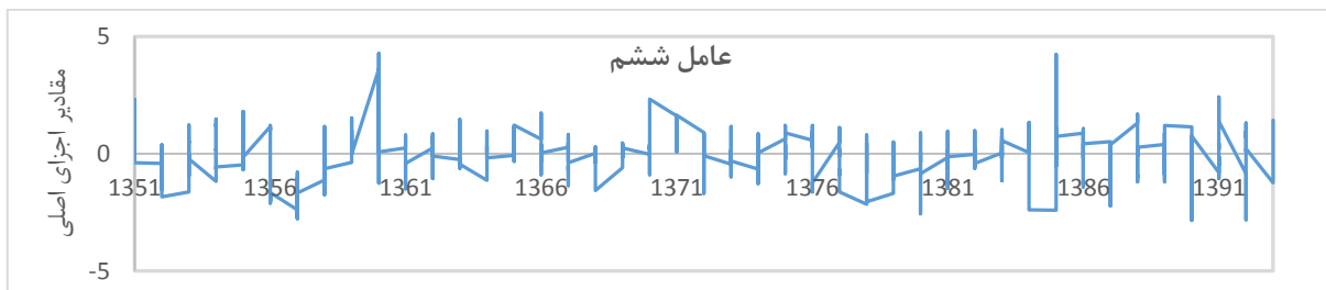
شکل ۴: مقادیر اجزای اصلی SPI سه ماهه استان گلستان
