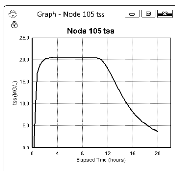
شکل (۴): کاهش غلظت جامدات معلق در سناریو ۴
