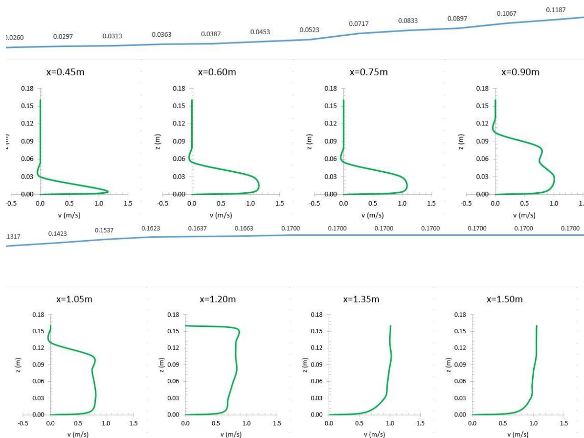
شکل (10): نیمرخ سرعت قائم در طول پرش هیدرولیکی در ۸ ایستگاه طولی مختلف در طی پرش هیدرولیکی با عرض نسبی ۰/۲ و عمق اولیه پرش هیدرولیکی ۰/۰۳۴ متر
