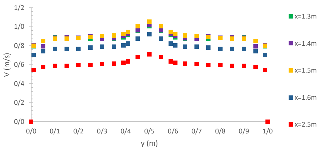
شکل (۱۱): نیمرخ سرعت طولی جریان در عرض مقطع مرکب در طی پرش هیدرولیکی با عرض نسبی ۰/۲ و عمق اولیه پرش هیدرولیکی ۰/۰۳۴ (متر)
