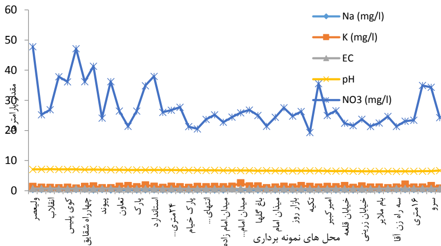
شکل (۳): تغییرات غلظت نیترات، سدیم، پتاسیم، EC و pH در آب شرب شهر ملایر
