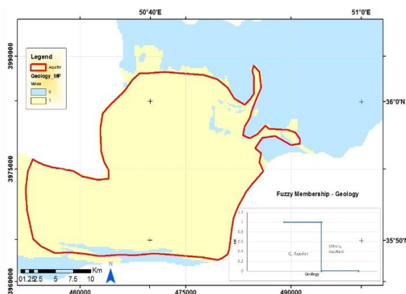
شکل (۳): تابع عضویت تعریف شده برای واحدهای آبرفت و سازند سخت و لایه رستر حاصل از تابع عضویت اعمال شده
