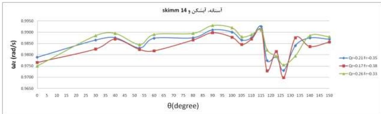
شکل ۱۱ - تغییرات مقدار چرخش جریان در طول قوس ۱۸۰ برای آزمایش آستانه، آبشکن و دیوار جداکننده ۱۴ درجه
