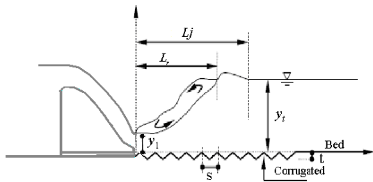
شکل (۱): چگونگی تشکیل پرش هیدرولیکی بر روی بستر با زبری‌های مثلی
