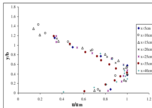
شکل (۴): پروفیل‌های بی‌بعد سرعت آزمایش B-۵
