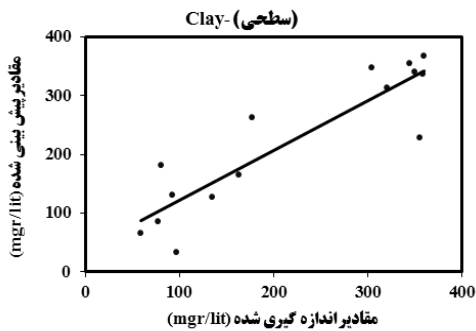
شکل ۳- مقایسه مقادیر اندازه‌گیری شده و مقادیر شبیه‌سازی شده توسط مدل شبکه عصبی مصنوعی برای نترات در سیستم آبیاری قطره‌ای سطحی
