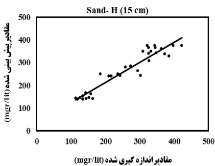
شکل ۴- مقایسه مقادیر اندازه گیری شده و مقادیر شبیه سازی شده توسط مدل شبکه عصبی مصنوعی برای نترات در سیستم آبیاری قطره‌ای سطحی
