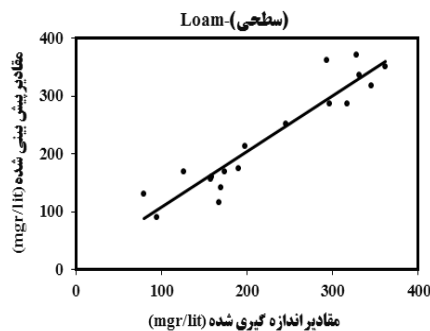
شکل ۳- مقایسه مقادیر اندازه‌گیری شده و مقادیر شبیه‌سازی شده توسط مدل شبکه عصبی مصنوعی برای نترات در سیستم آبیاری قطره‌ای سطحی
