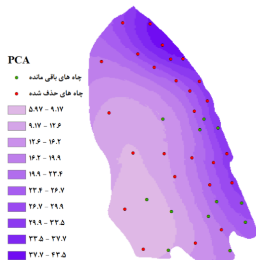
شکل ۴: چاه‌های حذف شده و باقی‌مانده در روش PCA
