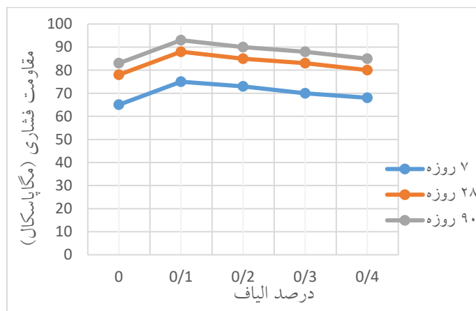
شکل (۶): نمودار تغییرات مقاومت فشاری نمونه‌های ۷، ۲۸ و ۹۰ روزه به ازاء درصد الیاف
