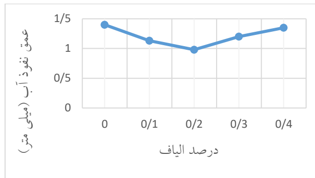
شکل (۱۰): نمودار تغییرات عمق نفوذ آب نمونه های بتنی به ازاء درصد الیاف
