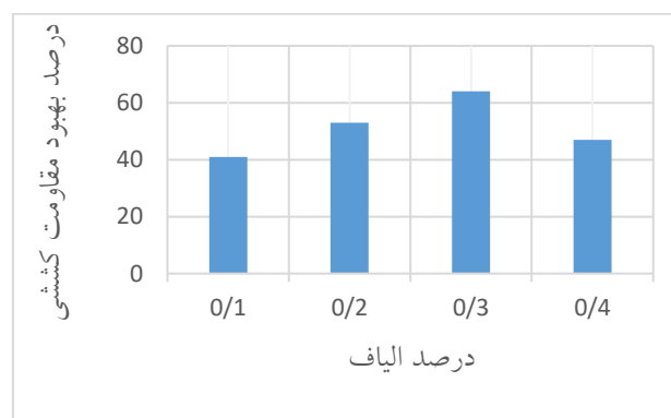
شکل (۹): نمودار درصد بهبود مقاومت کششی نمونه های بتنی به ازاء درصد الیاف، نسبت به نمونه‌های مرجع
