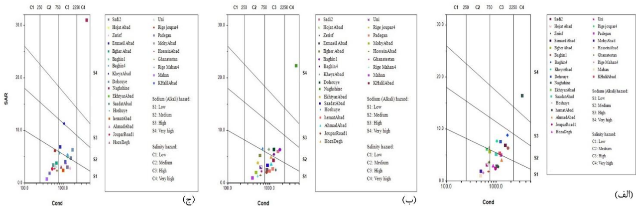
شکل (۱۲): ارزیابی کیفی آب دشت کرمان با توجه به نمودار ویلکاکس در سال‌های الف (۱۳۸۱)، ب (۱۳۹۲) و ج (۱۴۰۳)
