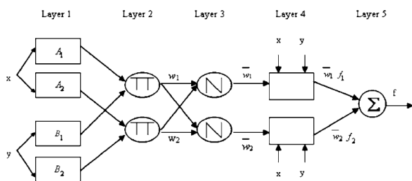
شکل (۲): شمایی از الگوریتم ANFIS
