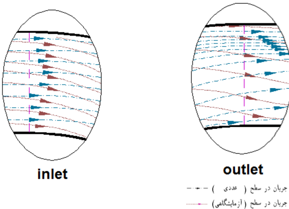
شکل (۹): بردارهای شبیه سازی شده خطوط جریان در محل ورودی و خروجی لوله زهکش
