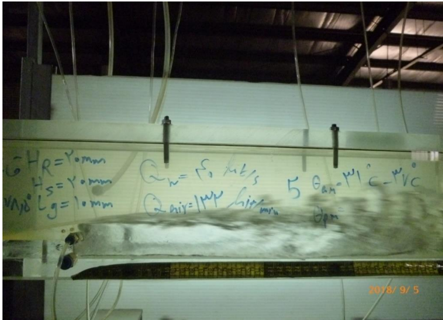
شکل (۳): ترکیب رمپ و پله و شکاف افقی با زاویه رأس 78/5^\circ تحت دبی آب 40 \text{ lit/s} به همراه هوادهی
