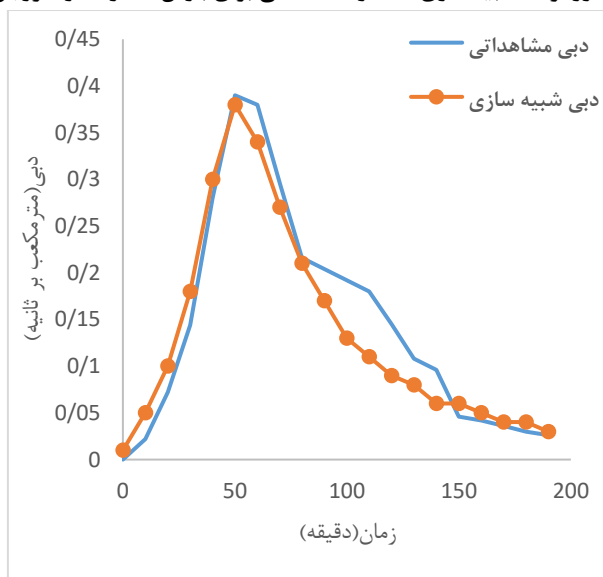
شکل (۷) هیدروگراف شبیه‌سازی شده و مشاهده‌ای برای بارش شماره ۲ و خروجی شماره ۲
