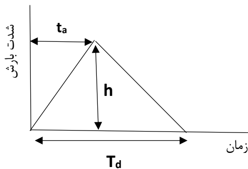
شکل (۳) روش هایتوگراف مثلثی
