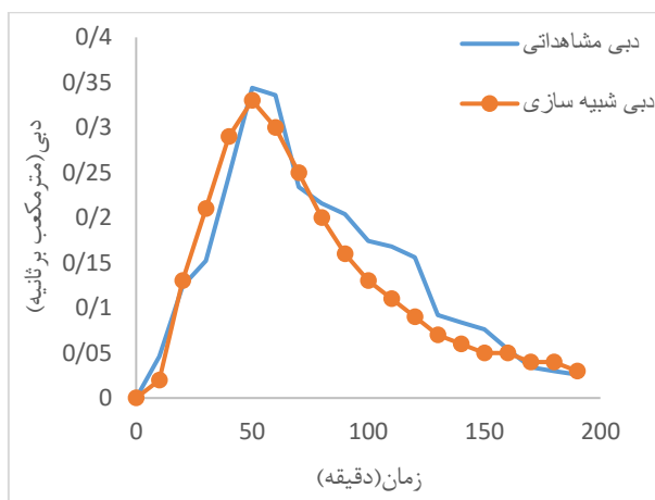
شکل (۷) هیدروگراف شبیه‌سازی شده و مشاهده‌ای برای بارش شماره ۲ و خروجی شماره ۲
