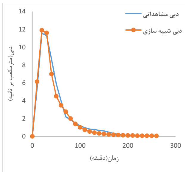
شکل (۹) هیدروگراف شبیه‌سازی شده و مشاهداتی برای بارش شماره ۴ و خروجی شماره ۲ جدول (۸) شاخص‌های آماری مرحله اعتبارسنجی برای خروجی شماره یک
