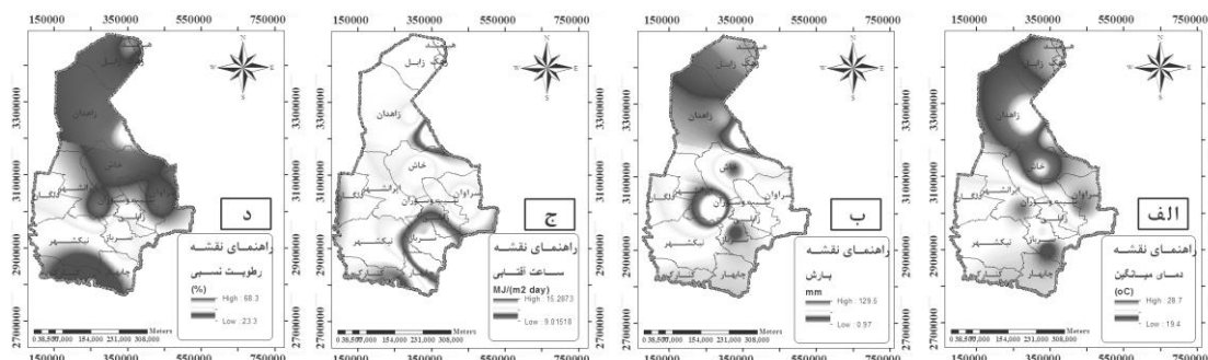
شکل (۲): پراکنش مکانی مقادیر (الف) متوسط دمای میانگین سالانه، (ب) بارش، (ج) تابش و (د) رطوبت نسبی در
