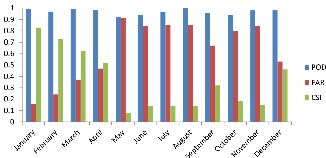
شکل (۳): مقایسه داده های بارش ماهواره ای و زمینی براساس شاخص های POD، FAR و CSI در مقیاس ماهانه
