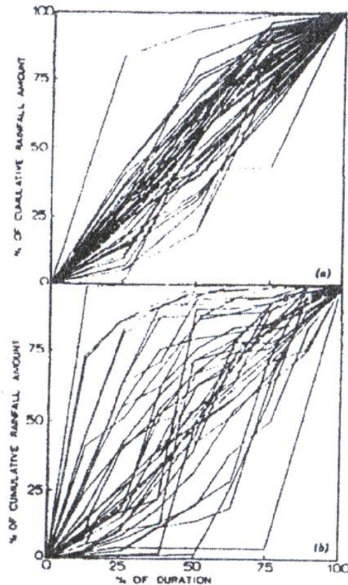
شکل (۱): منحنی تجمعی متوسط رگبارهای ۲۰ دقیقه (a) و ۴ ساعته (b)
