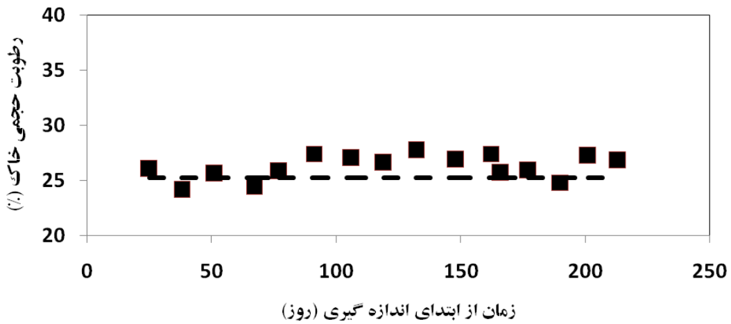
شکل (5): مقایسه رطوبت خاک قبل از آبیاری در تیمار آبیاری 80٪ در سال دوم با خط رطوبت بحرانی
