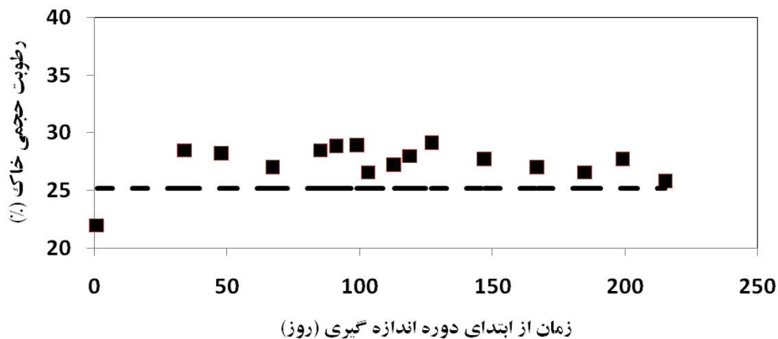
شکل (2): مقایسه رطوبت خاک قبل از آبیاری در تیمار آبیاری 80٪ در سال اول با خط رطوبت بحرانی
