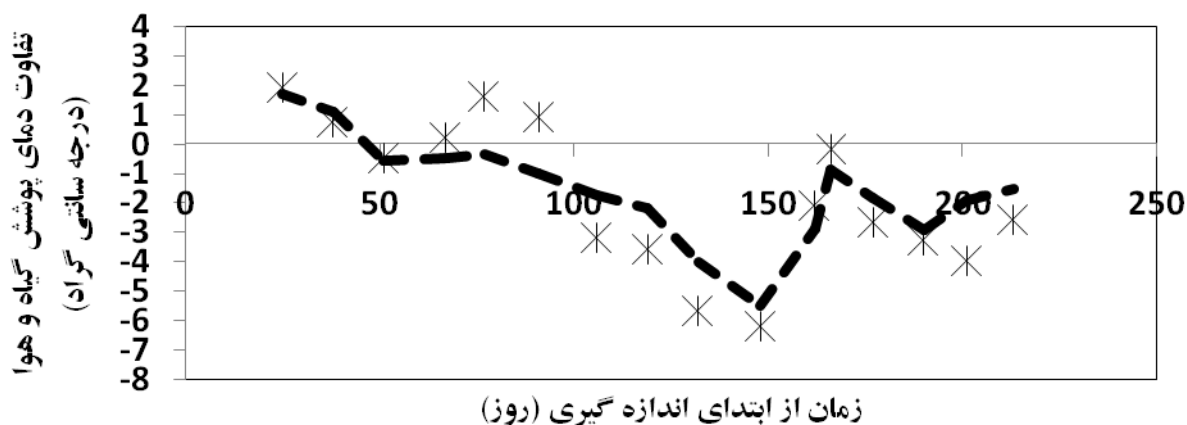
شکل (12): مقایسه تفاوت دمای گیاه و دمای هوا در تیمار شاهد در سال دوم با خط مقدار بحرانی
