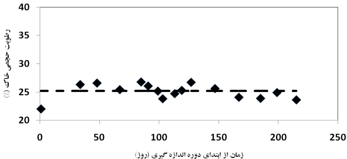
شکل (1): مقایسه رطوبت خاک قبل از آبیاری در تیمار آبیاری 60٪ در سال اول با خط رطوبت بحرانی
