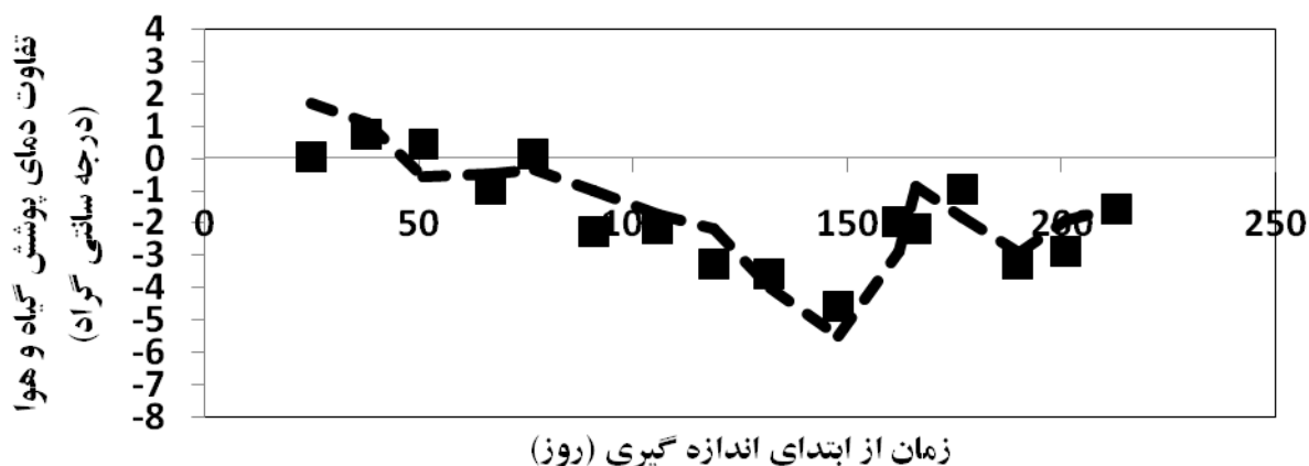
شکل (11): مقایسه تفاوت دمای گیاه و دمای هوا در تیمار آبیاری 80٪ در سال دوم با خط مقدار بحرانی
