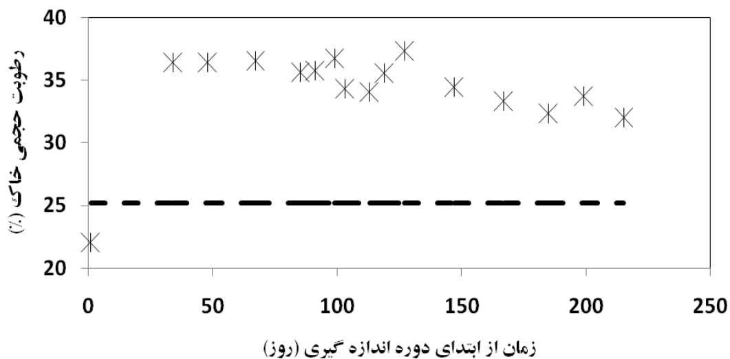
شکل (3): مقایسه رطوبت خاک قبل از آبیاری در تیمار شاهد در سال اول با خط رطوبت بحرانی
