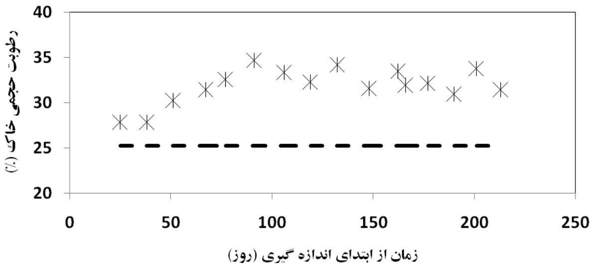
شکل (6): مقایسه رطوبت خاک قبل از آبیاری در تیمار شاهد در سال دوم با خط رطوبت بحرانی
