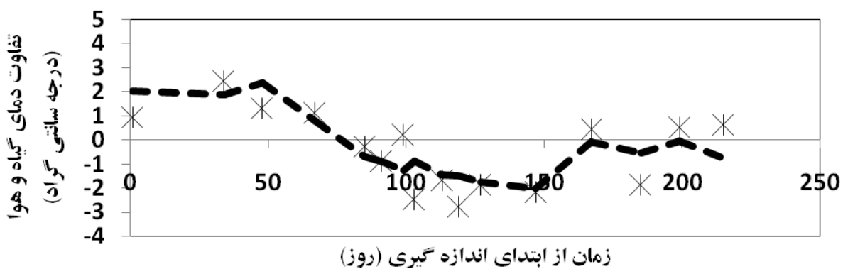
شکل (9): مقایسه تفاوت دمای گیاه و دمای هوا در تیمار شاهد در سال اول با خط مقدار بحرانی
