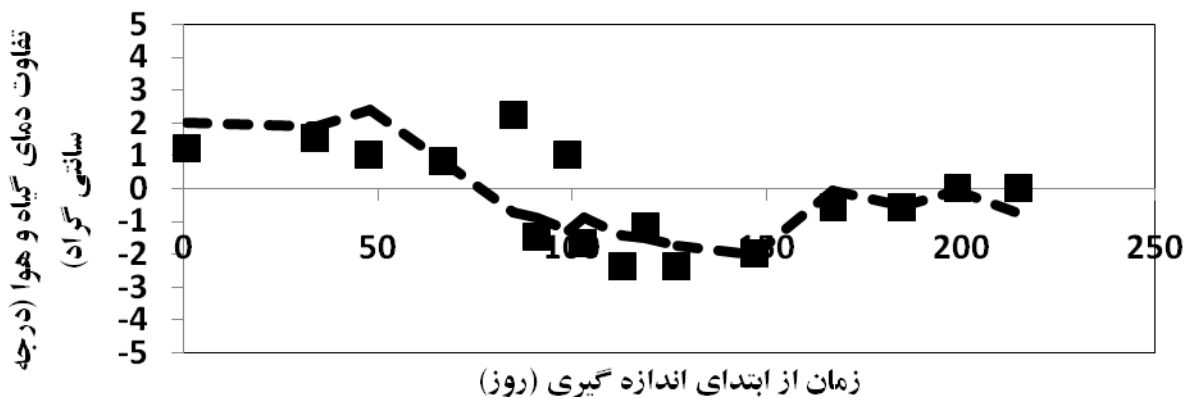
شکل (8): مقایسه تفاوت دمای گیاه و دمای هوا در تیمار آبیاری 80% در سال اول با خط مقدار بحرانی
