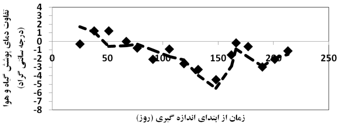
شکل (10): مقایسه تفاوت دمای گیاه و دمای هوا در تیمار آبیاری 60% در سال دوم با خط مقدار بحرانی
