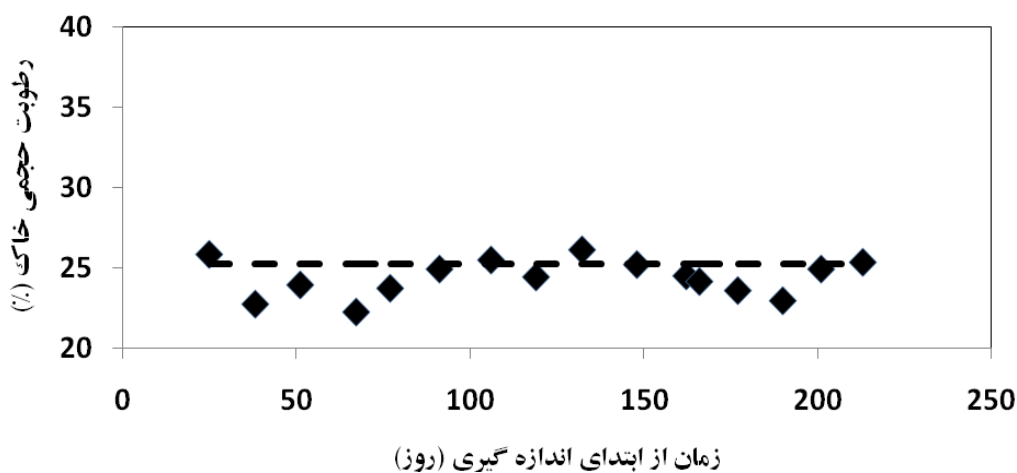
شکل (4): مقایسه رطوبت خاک قبل از آبیاری در تیمار آبیاری 60٪ در سال دوم با خط رطوبت بحرانی
