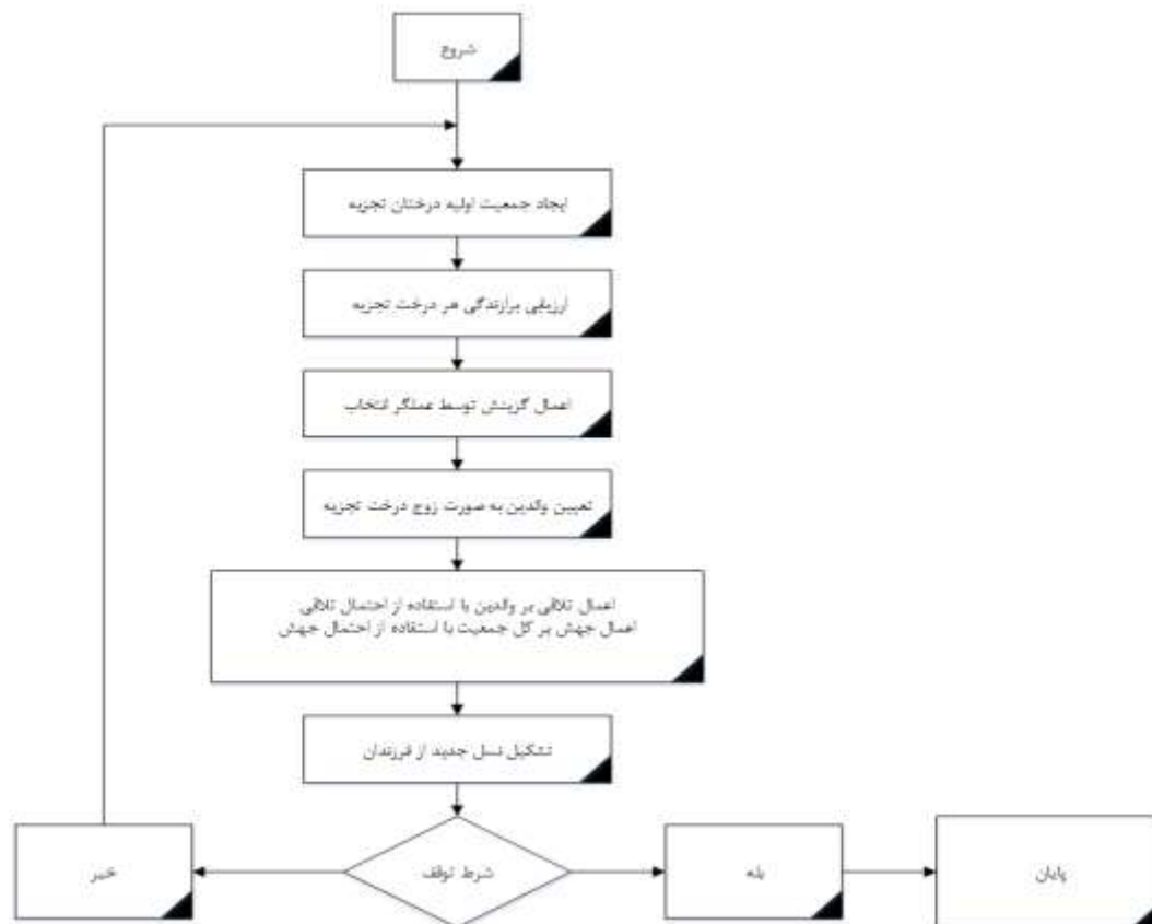
شکل ۲- فلوچارت مدل برنامه‌ریزی ژنتیک.
