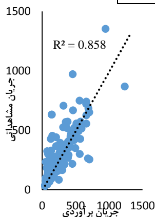
شکل ۵- مقایسه نتایج مدل برنامه‌ریزی بیان ژن با مقادیر مشاهده‌ای، مرحله تست.
