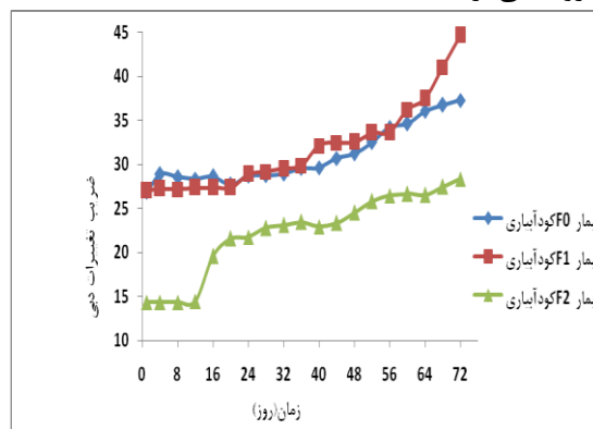
شکل (۴): تأثیر غلظت‌های مختلف کود آبیاری بر ضریب تغییرات دبی قطره‌چکان‌های C
