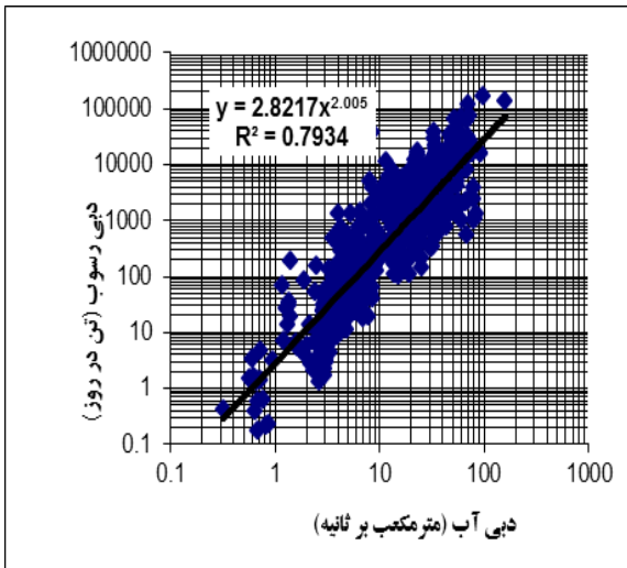
شکل (۵): منحنی سنجه رسوب یک خطی ایستگاه گلینیک
