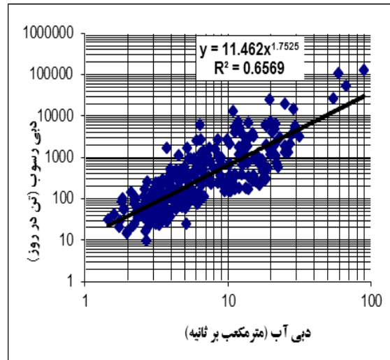
شکل (۴): منحنی سنجه رسوب یک خطی ایستگاه باغکلایه
