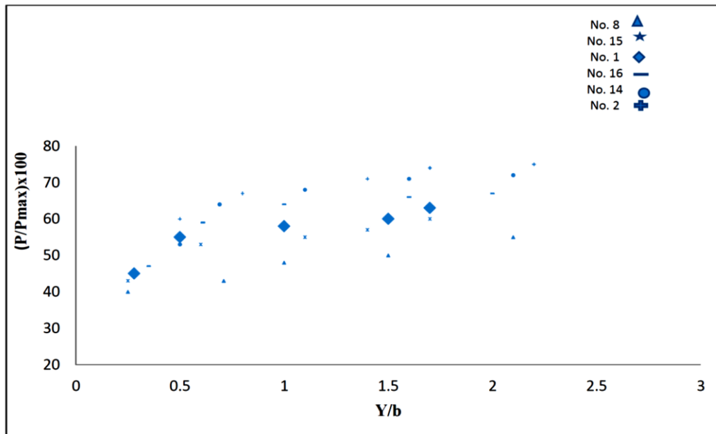
شکل (۱۲): نسبت درصد فشار حداکثر در مقابل تغییرات عمق نسبت به عرض در مدل‌های شماره‌ی ۸، ۱۵، ۱۶، ۱، ۱۴، ۲.
