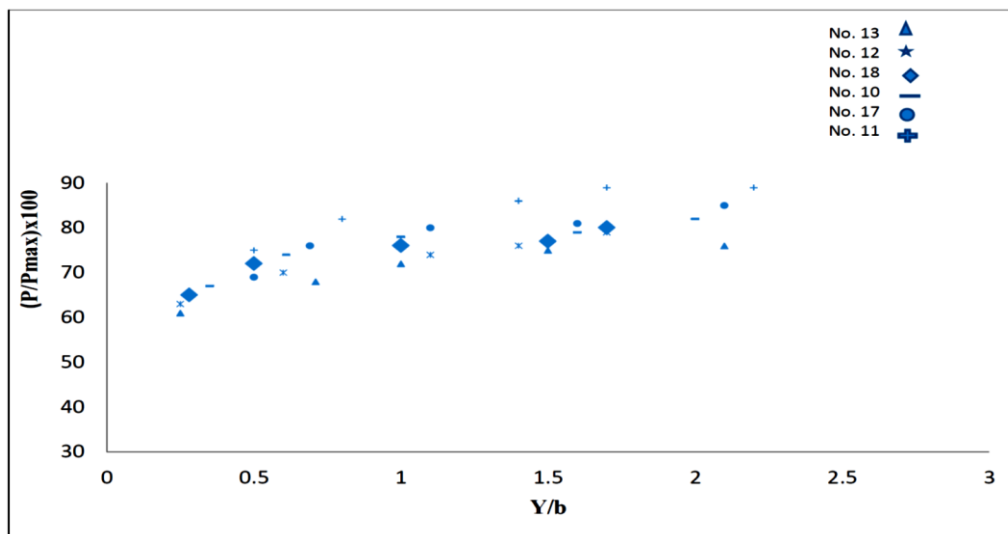
شکل (۱۳): نسبت درصد فشار حداکثر در مقابل تغییرات عمق نسبت به عرض در مدل‌های شماره‌ی ۱۱، ۱۲، ۱۰، ۱۸، ۱۷، ۱۳.
