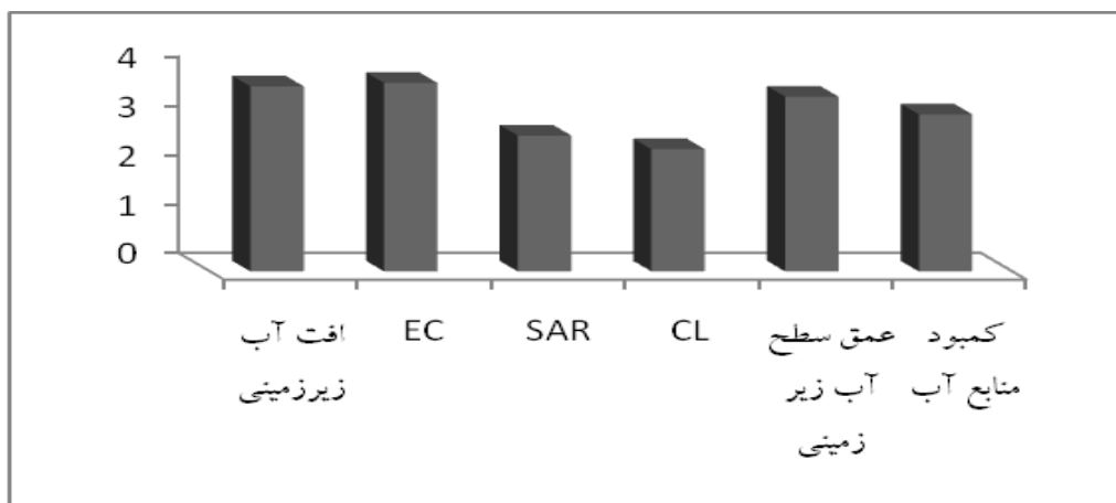
شکل (۱): متوسط وزنی ارزش‌های کمی شاخص‌های موثر بر معیار آب زیرزمینی
