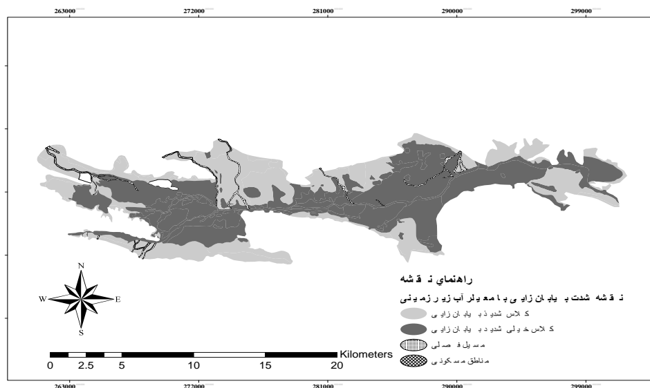
شکل (۳): شدت بیابان‌زایی از جنبه معیار آب منطقه‌ای مزایجان
